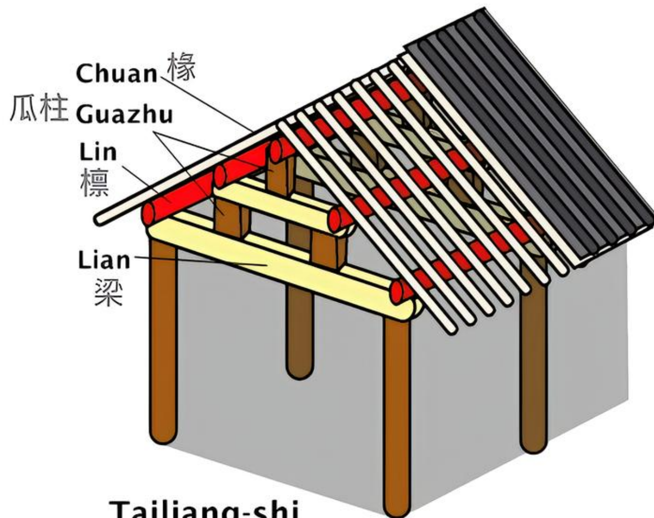
抬梁式
